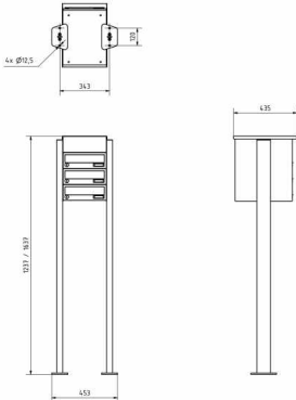
Montagebohrungen
