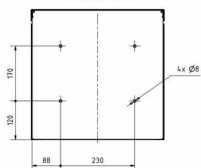
Montagebohrungen
