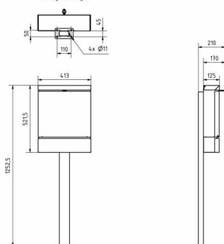
Montagebohrungen
