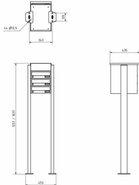
Front-ansichten
