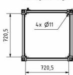
Montagebohrungen
