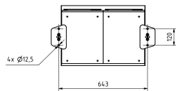
Montagebohrungen
