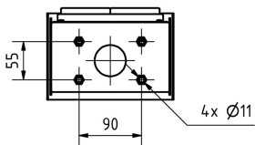
Montagebohrungen
