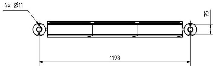
Montagebohrungen
