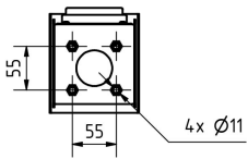
Montagebohrungen
