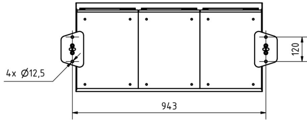
Montagebohrungen
