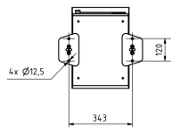
Montagebohrungen
