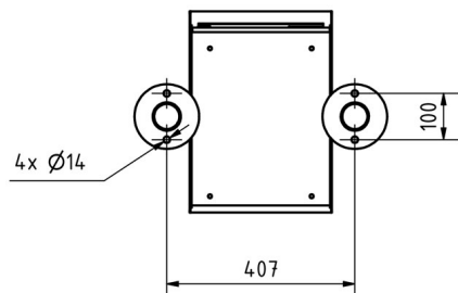
Montagebohrungen
