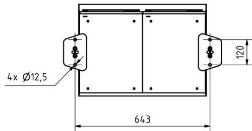
Montagebohrungen
