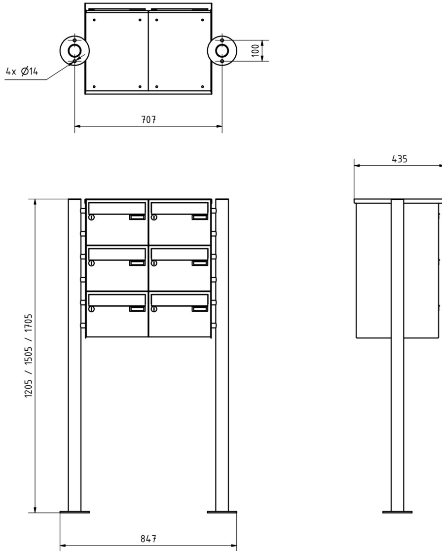
Montagebohrungen
