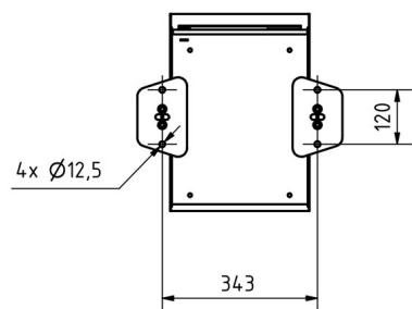
Montagebohrungen
