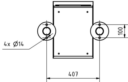
Montagebohrungen
