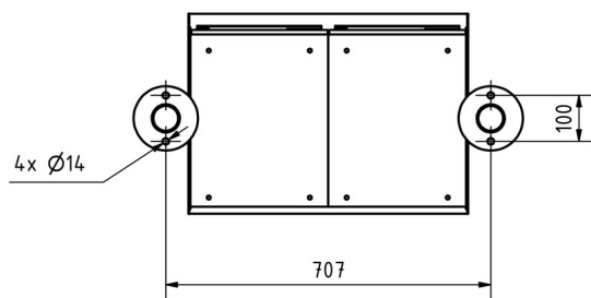
Montagebohrungen
