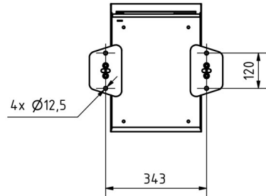
Montagebohrungen
