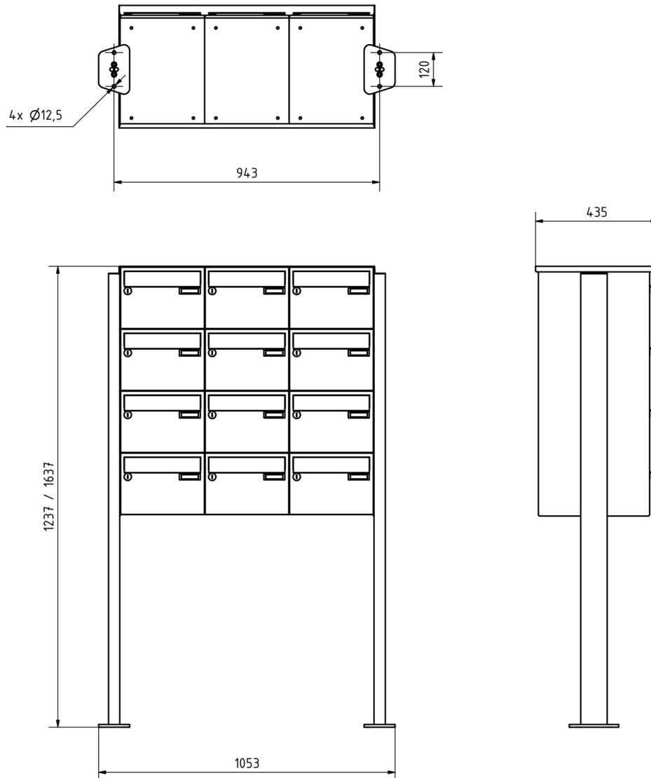
Montagebohrungen
