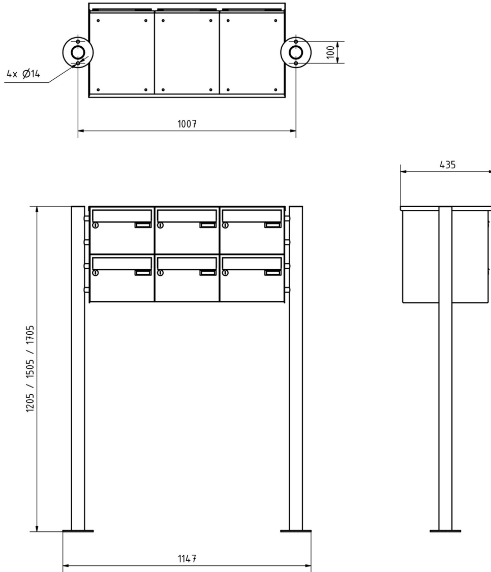
Montagebohrungen
