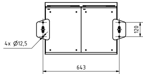
Montagebohrungen
