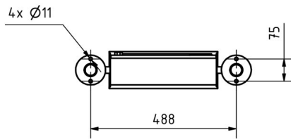
Montagebohrungen
