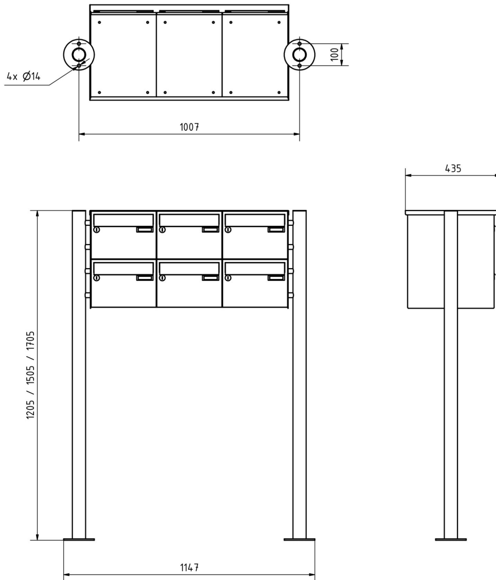
Montagebohrungen
