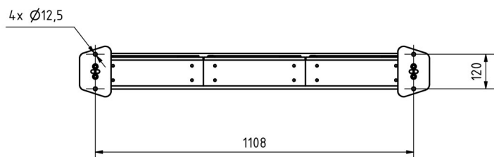
Montagebohrungen
