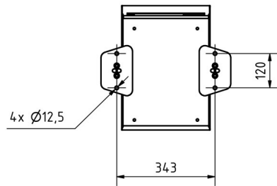
Montagebohrungen
