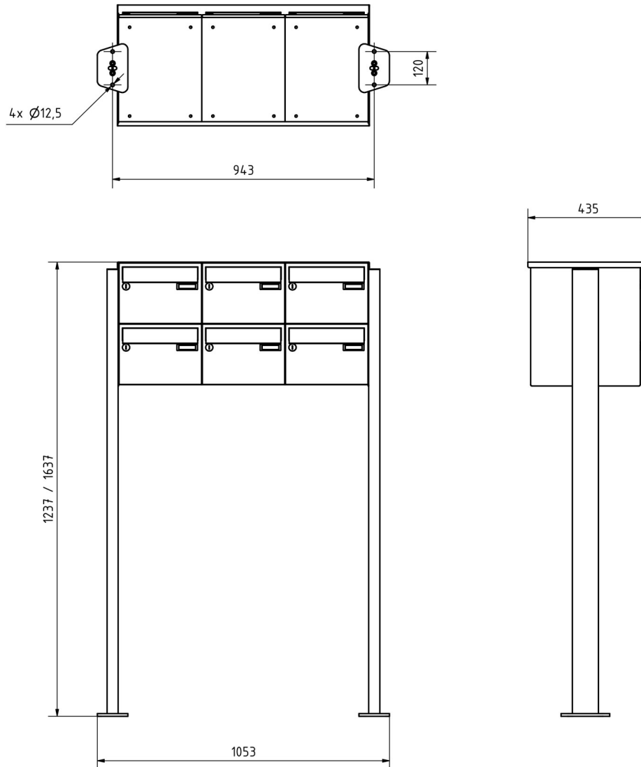
Montagebohrungen
