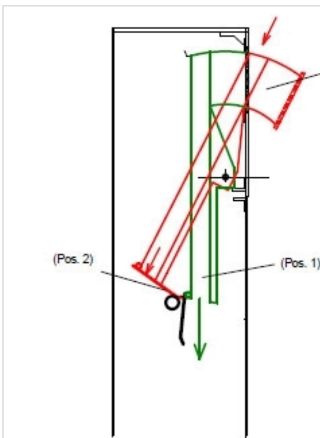
Prinzip der Schleusentechnik (gebrauchsmustergeschützt)
