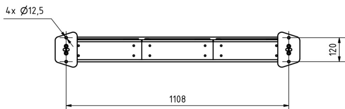
Montagebohrungen
