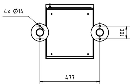
Montagebohrungen
