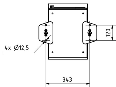
Montagebohrungen
