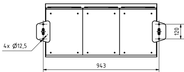
Montagebohrungen
