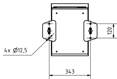
Montagebohrungen
