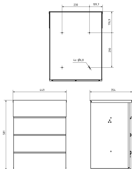
Montagebohrungen ( 1 : 5 )
