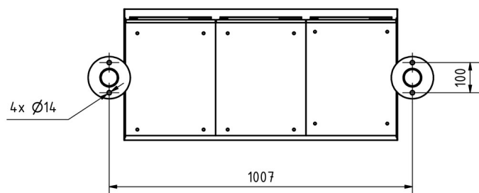
Montagebohrungen
