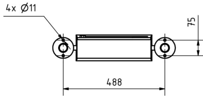
Montagebohrungen
