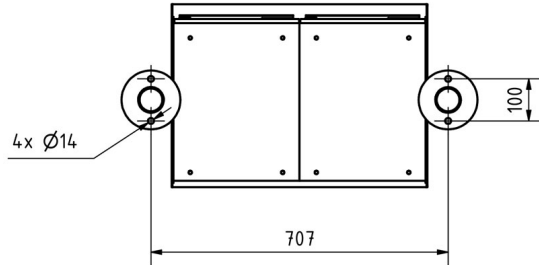
Montagebohrungen
