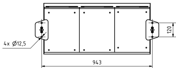
Montagebohrungen
