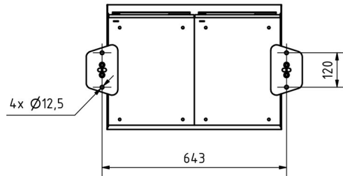
Montagebohrungen
