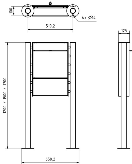
Montagebohrung
