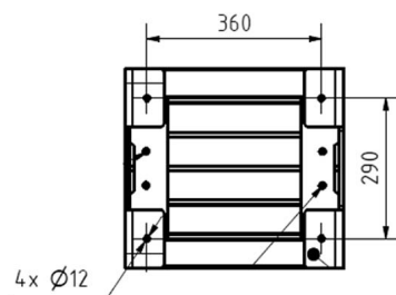
Bohrbild Bodenbefestigung
