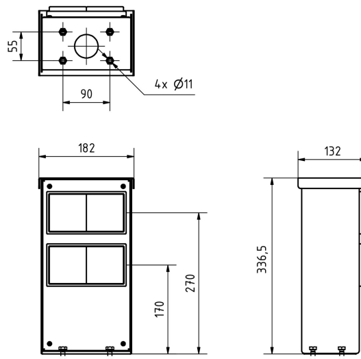
Montagebohrungen
