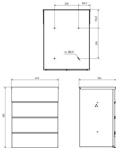
Montagebohrungen ( 1 : 5 )
