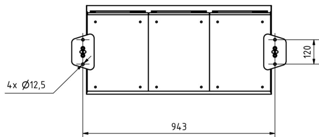
Montagebohrungen
