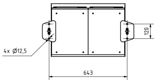
Montagebohrungen
