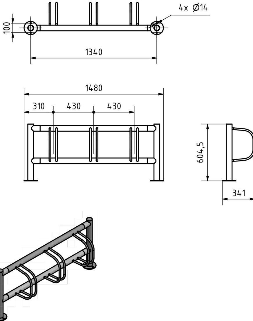
Montagebohrungen ( 1 : 20 )
