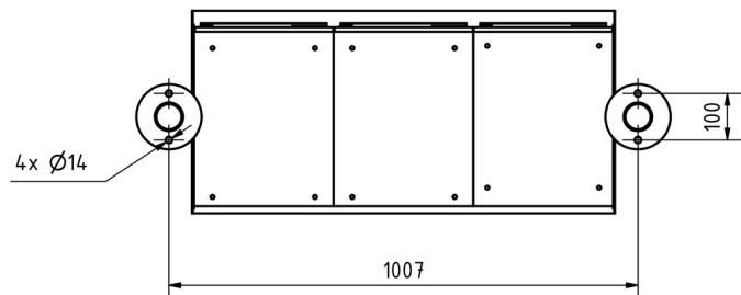
Montagebohrungen
