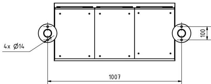
Montagebohrungen
