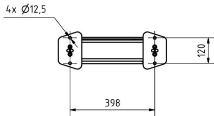
Montagebohrungen
