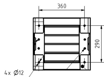
Bohrbild Bodenbefestigung
