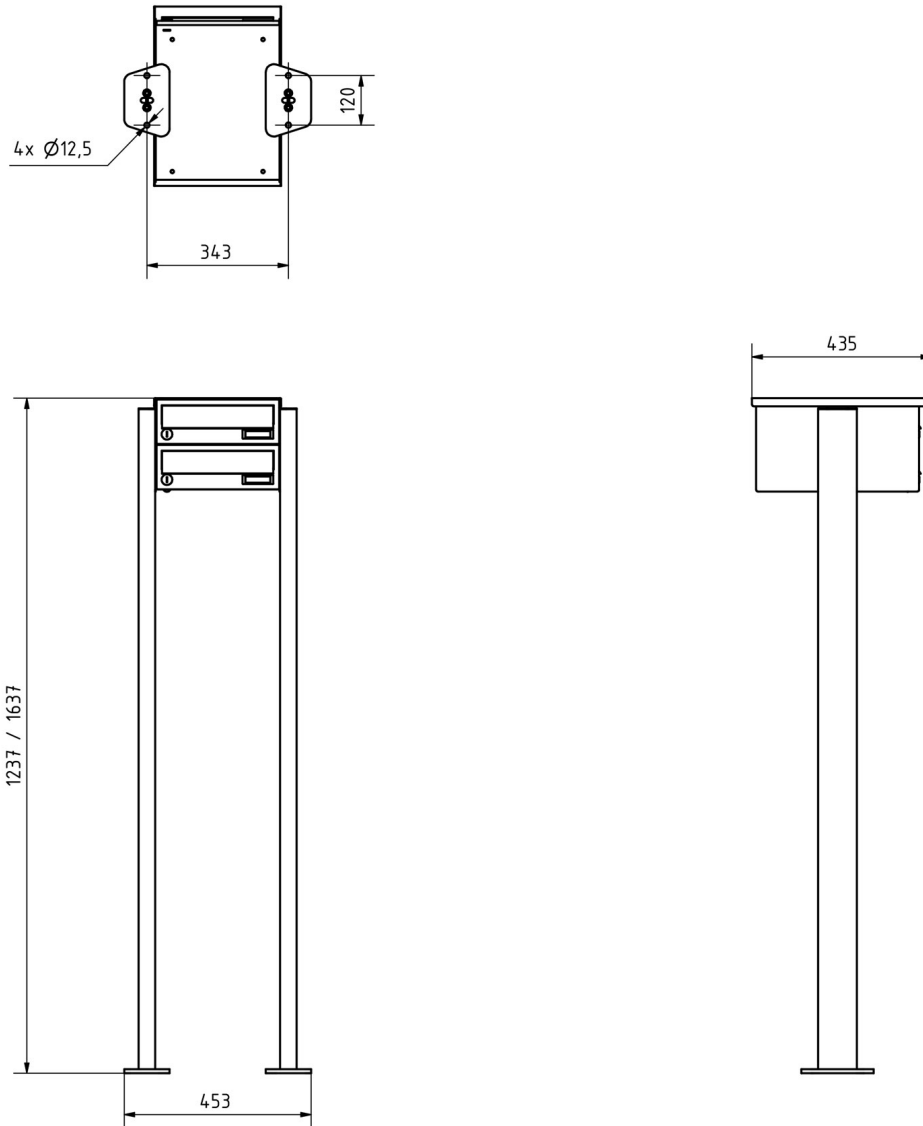
Montagebohrungen
